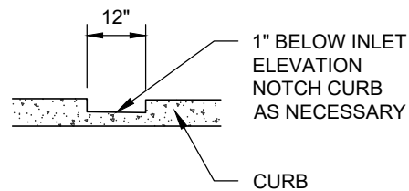
SECTION B-B - OUTLET OPENING N.T.S.
