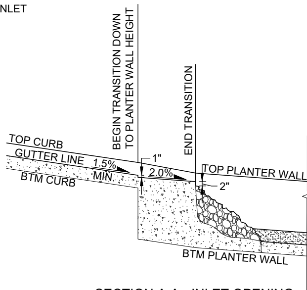
SECTION A-A - INLET OPENING N.T.S.
