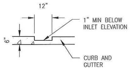
SECTION A-A OUTLET NOTCH N.T.S.
